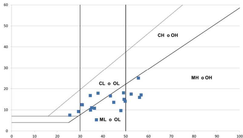
Figura 1. Representación de las muestras con plasticidad en el ábaco de Casagrande.
