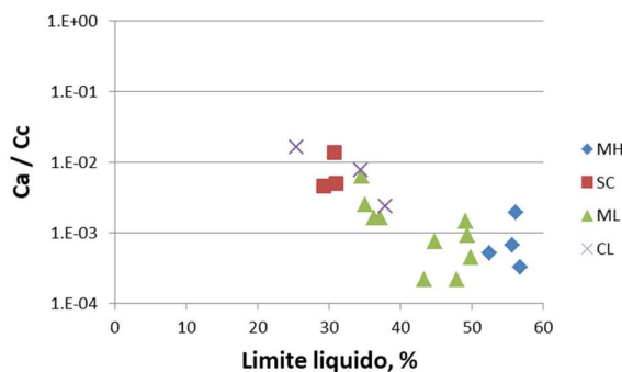
Figura 10. Relación C_a/C_c frente al límite líquido para las diferentes muestras analizadas
