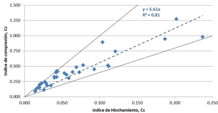
Figura 3. Relación C_c / C_s
