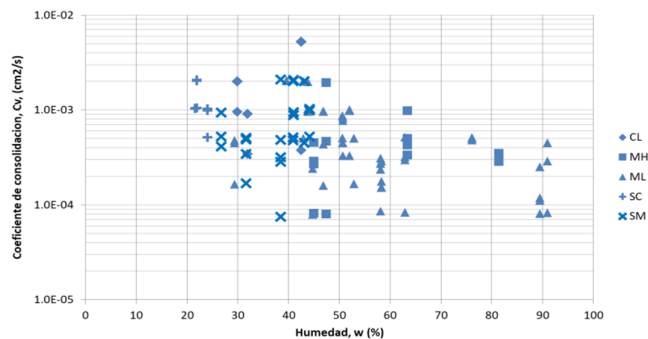
Figura 6. Representación gráfica C_v frente a w de las muestras analizadas
