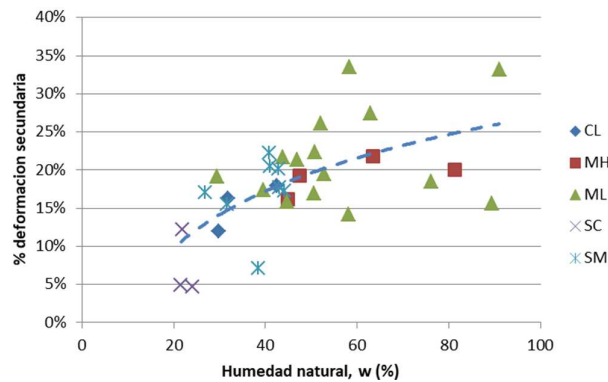
Figura 12. Proporción que supone la deformación secundaria frente a la humedad natural del material
