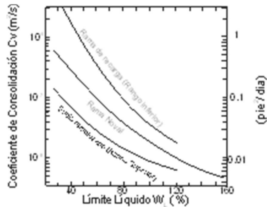
Figura 7. Correlación aproximada C_v – límite líquido. Fuente: Traducido de NAVFAC D.M. 7.01 (1986) [3]
