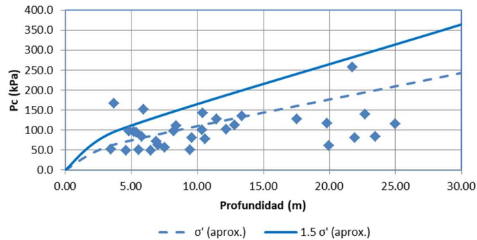
Figura 2. Presión de preconsolidación vs profundidad
