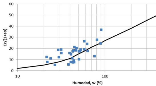
Figura 5. Relación C_c / 1+e_0 vs humedad propuesta por Lambe & Whitman (1969)
