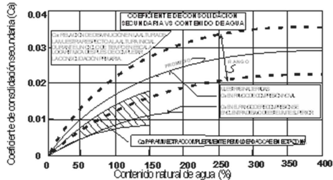
Figura 9. Correlación aproximada C_a – humedad. Fuente: Traducido de NAVFAC D.M. 7.01 (1986)
