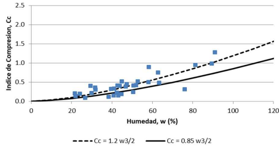
Figura 4. Relación índice de compresión vs humedad propuesta por Henelelund (1951) ajustada
