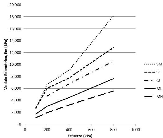
Figura 11. Evolución de los módulos edométricos en función de la carga aplicada
