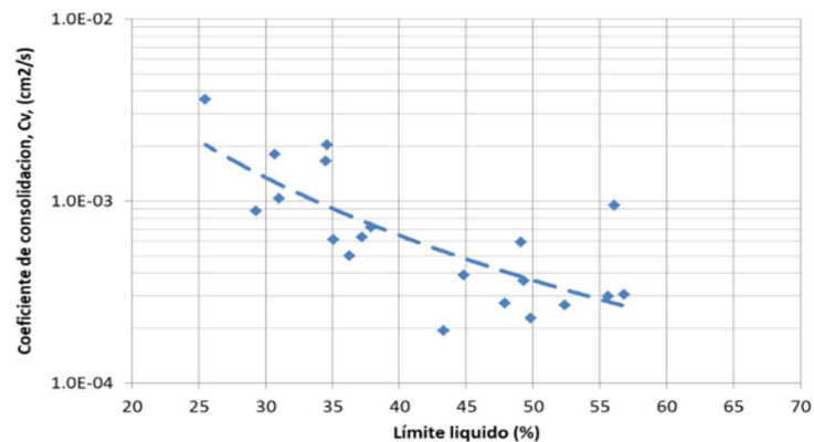
Figura 8. Representación resultados C_v (rama de consolidación noval) – límite líquido.
